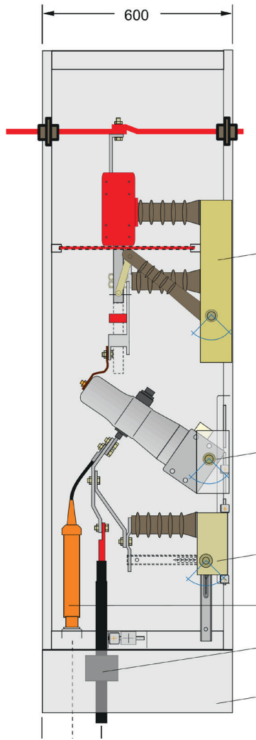
Festeinbau-Technik D-Feld, Frontansicht
