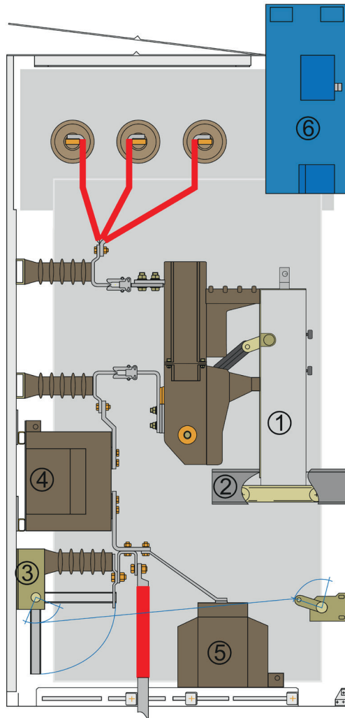
Einschub-Technik W-Feld, Seitenansicht
