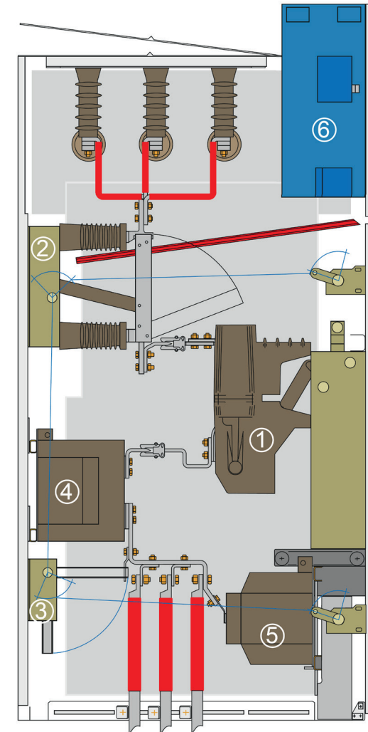
Mobile Festeinbau-Technik W-Feld, Seitenansicht
